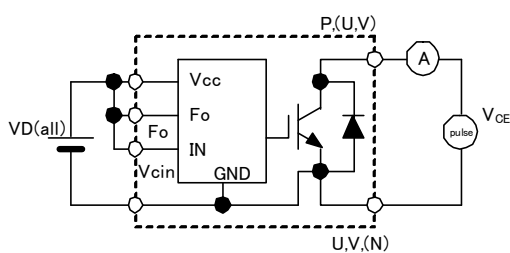
Fig. 5 I_{CES} Test
